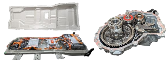
日産・サクラの分解部品
