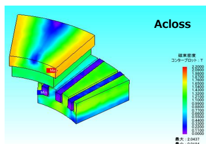
JMAGによる電磁場解析
