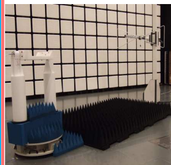
電波暗室/電磁波 評価システム
